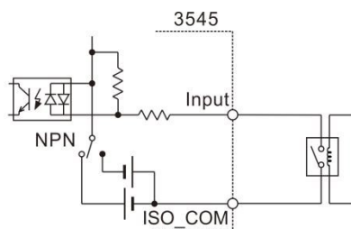
继电器输入
