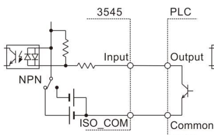
PLC的NPN输出
