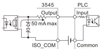
PLC 的 NP 输入
