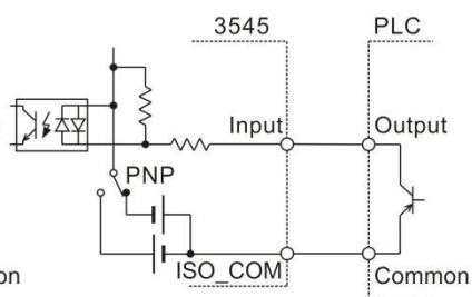
PLC的PNP输出
