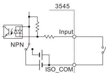
开关输入
