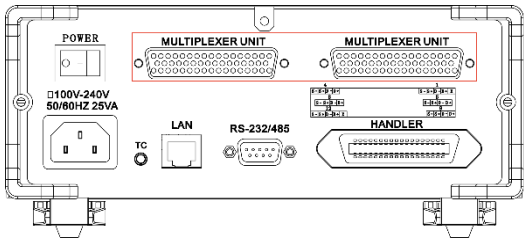
四线制测试端口
