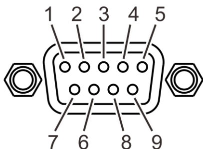
9-pin D-Sub 母口
