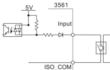
继电器输入
