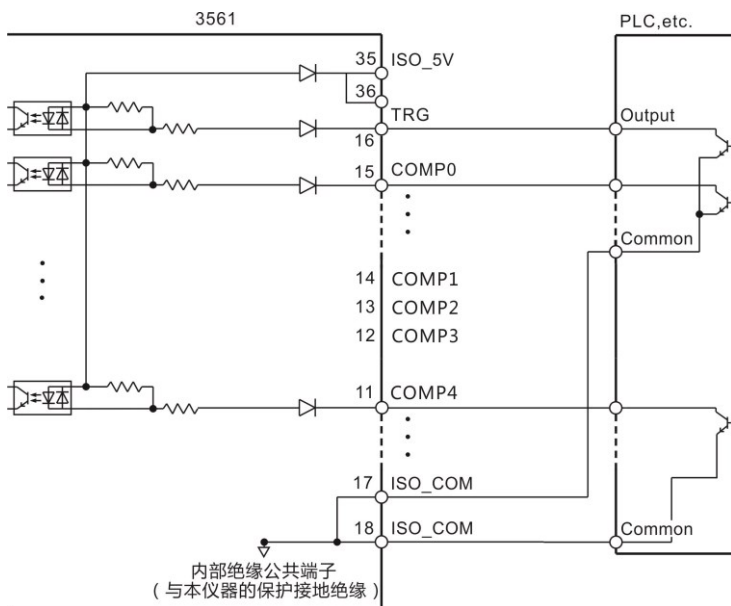
输出端原理图
