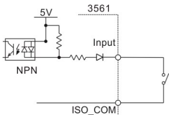
开关输入
